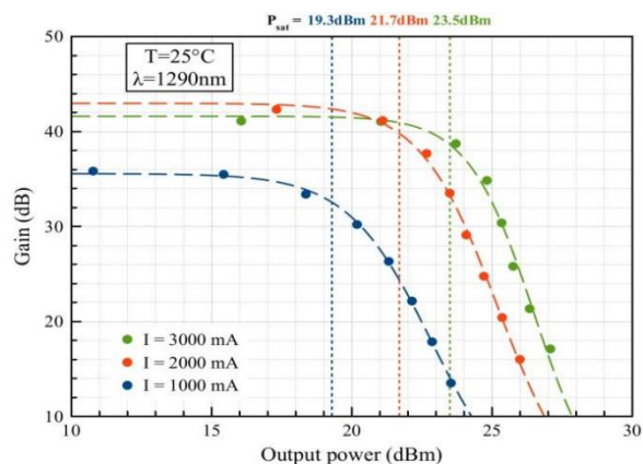
增益与输出功率
