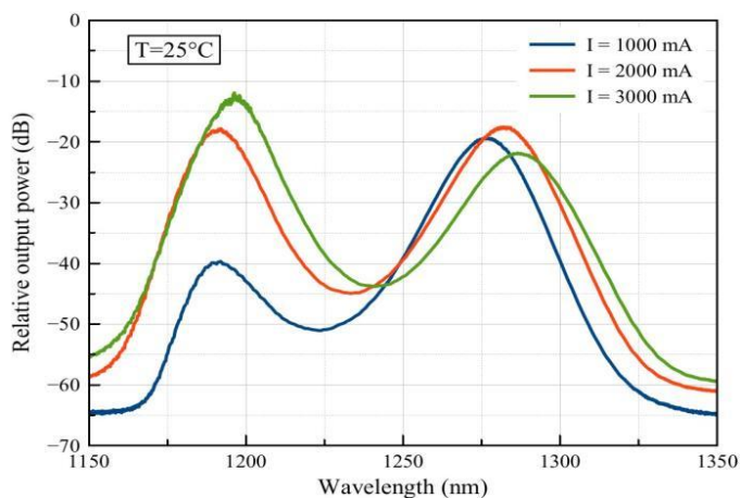
光谱(ASE)
