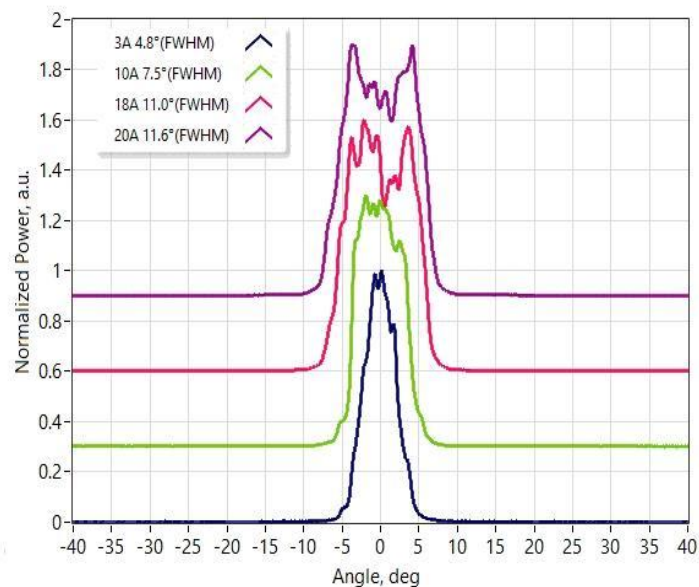
慢轴远场
