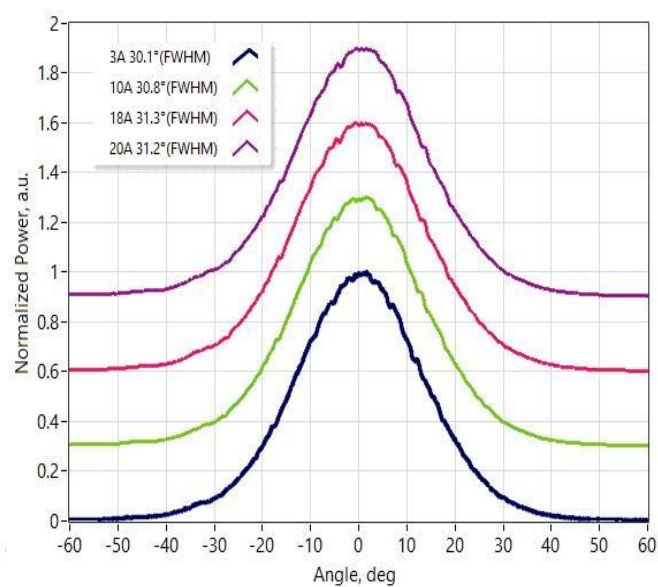
快轴远场
