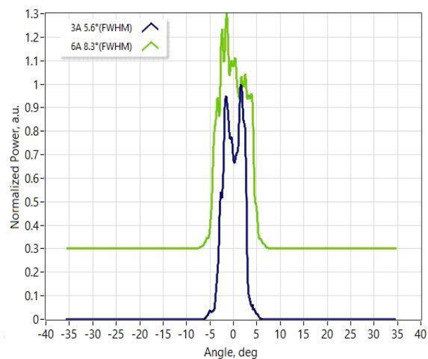
慢轴远场
