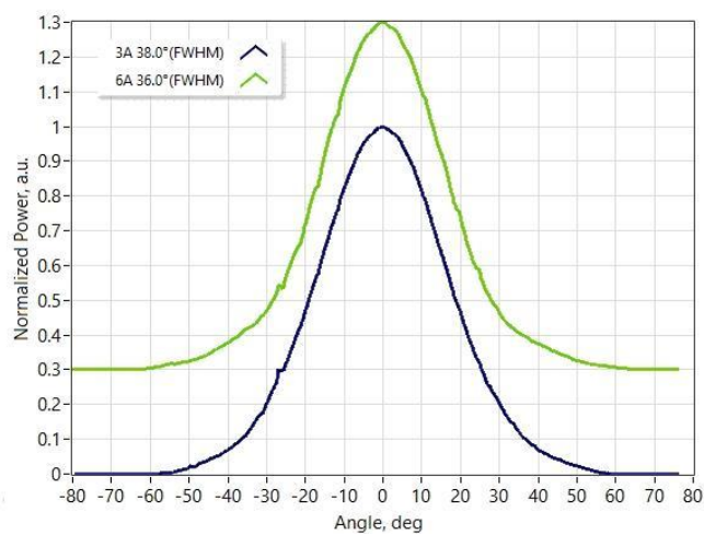
快轴远场
