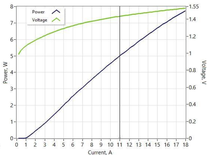
光-电流-电压特性
