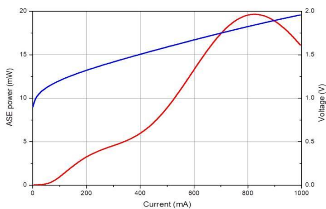
L-I-V 曲线
