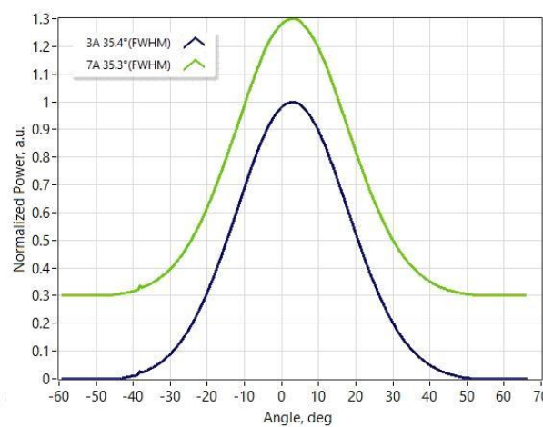
快轴远场
