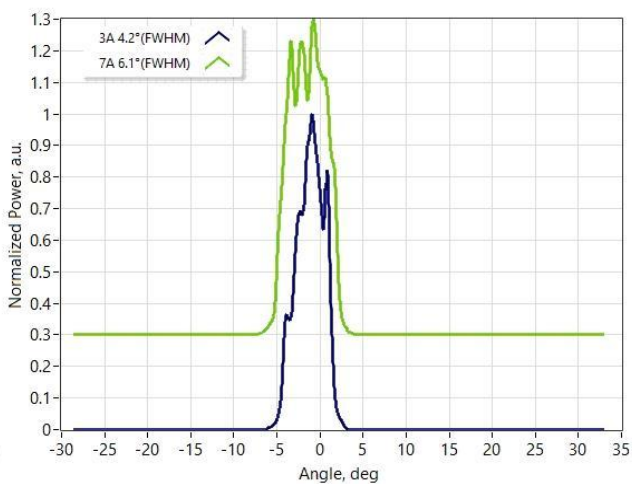
慢轴远场
