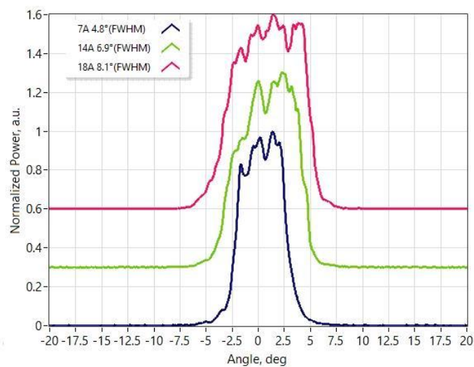
慢轴远场
