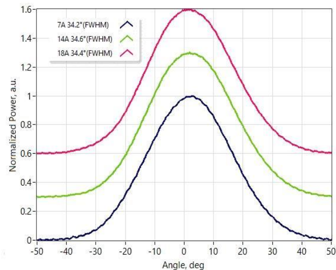
快轴远场
