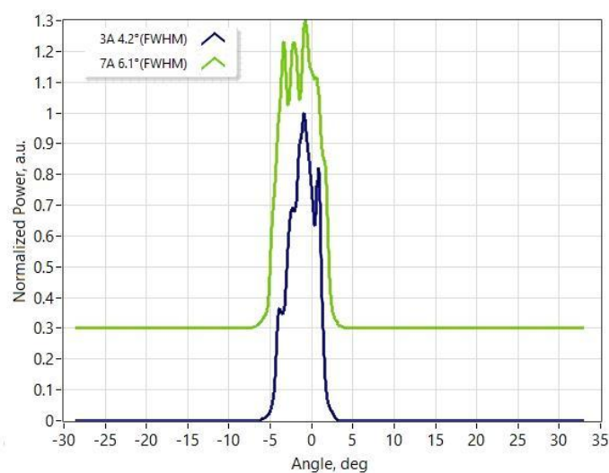
慢轴远场
