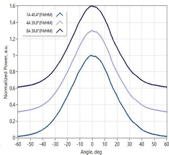
快轴远场
