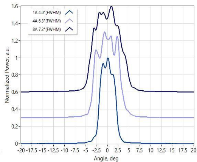
慢轴远场
