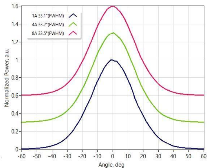
快轴远场
