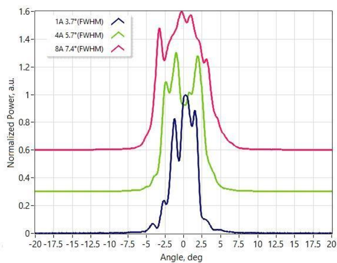
慢轴远场
