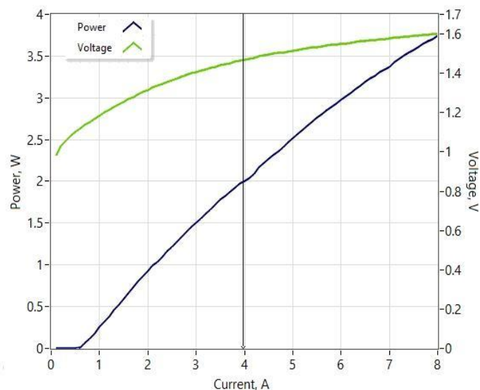
光-电流-电压特性
