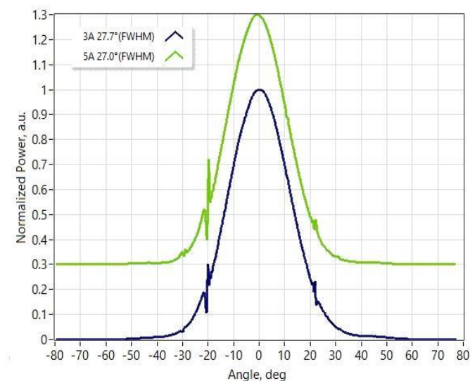
快轴远场
