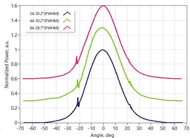
快轴远场
