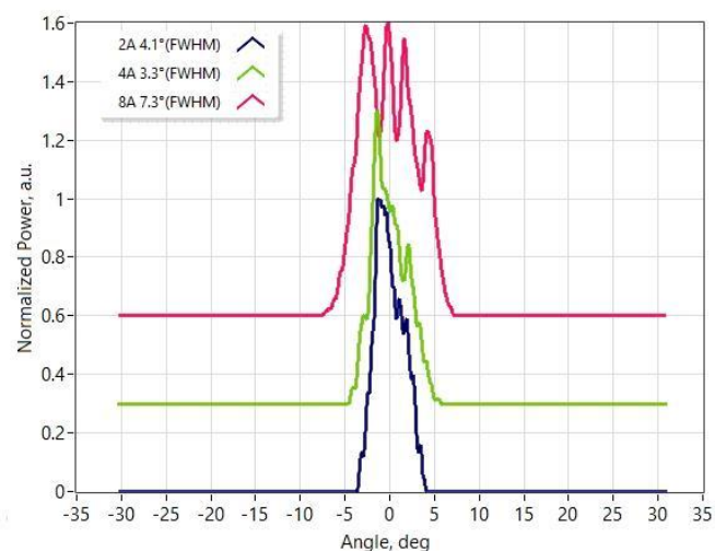
慢轴远场
