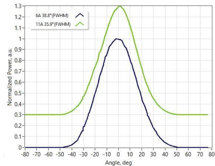
快轴远场
