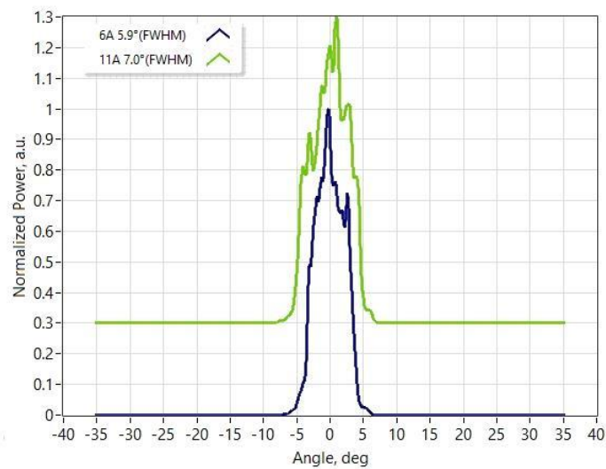
慢轴远场
