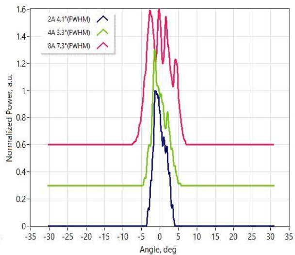
慢轴远场
