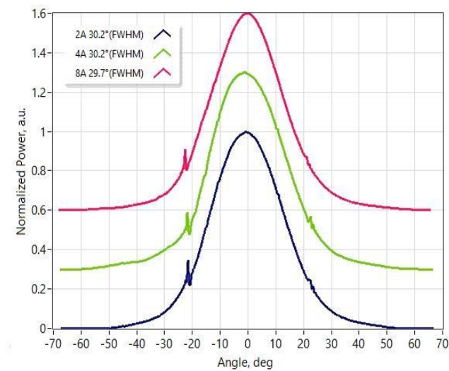
快轴远场
