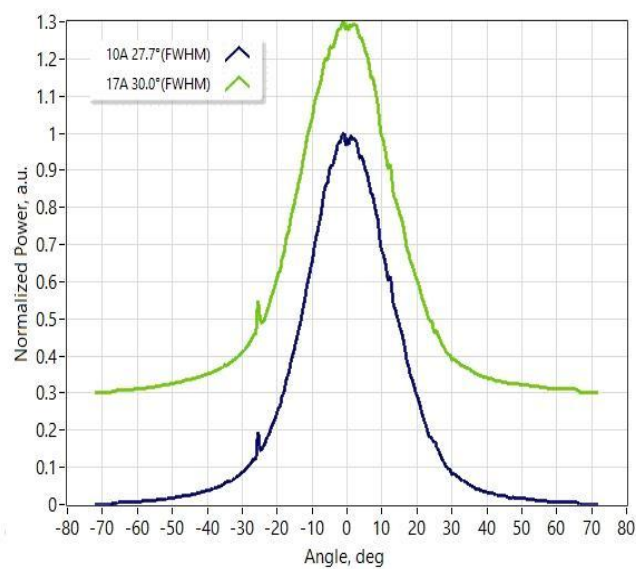
快轴远场
