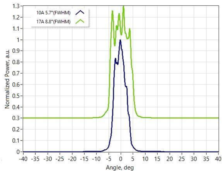
慢轴远场
