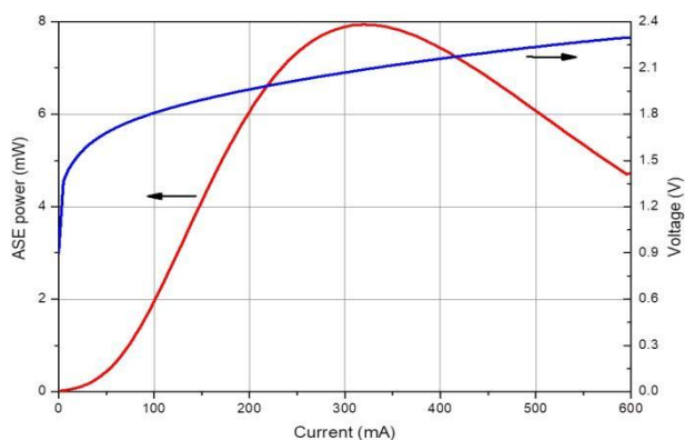
L-I-V 曲线
