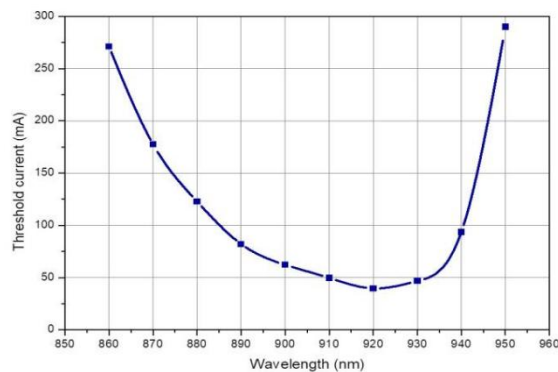
阈值电流
