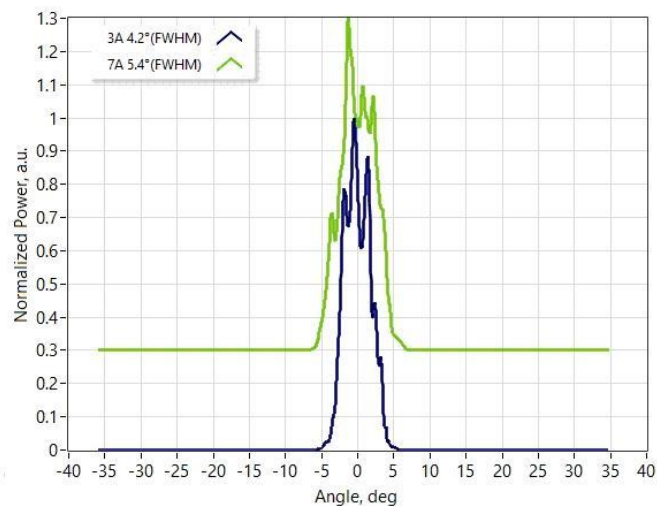
慢轴远场
