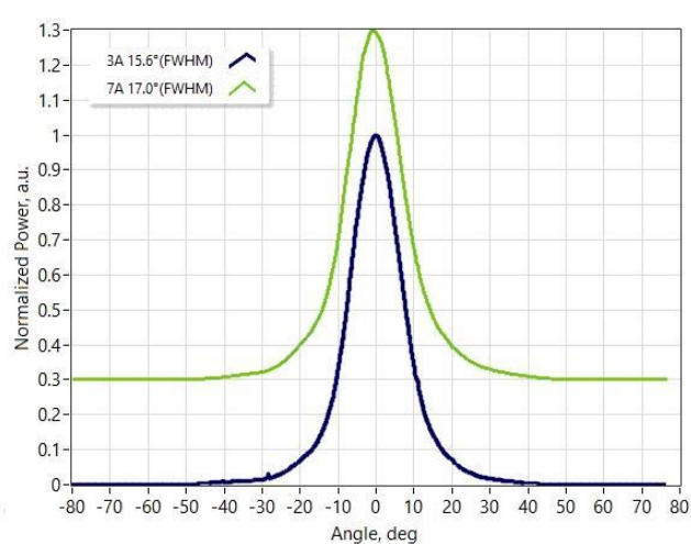
快轴远场
