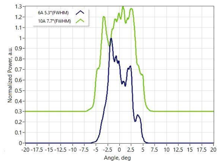
慢轴远场
