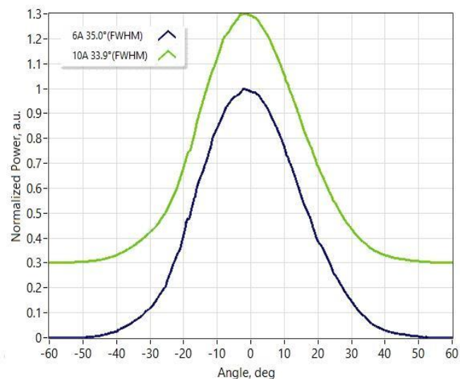
快轴远场
