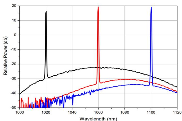
光谱(ASE)
