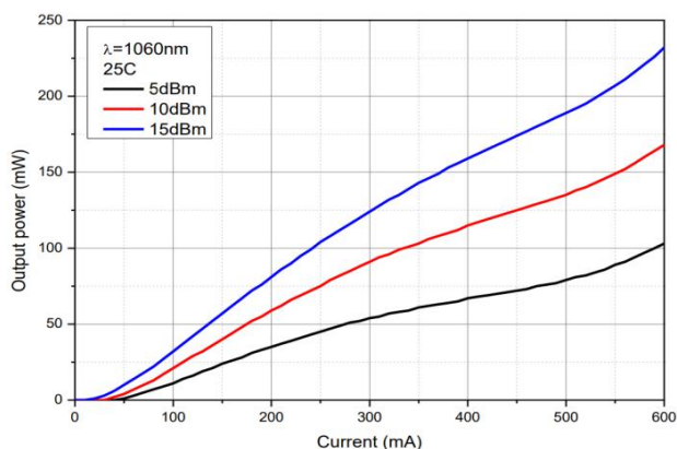
ASE LIV 特性
