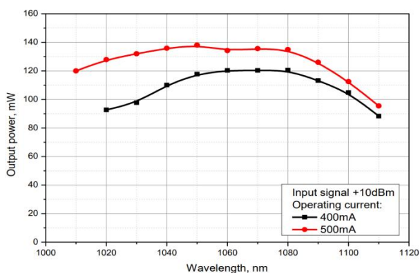
不同电流下的功率谱
