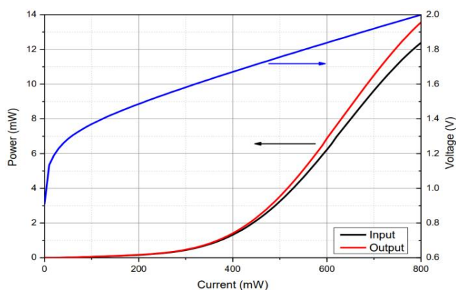
ASE LIV 特性
