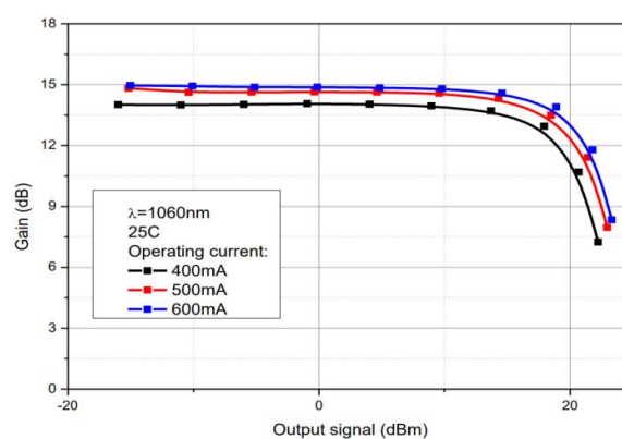
增益与输出功率
