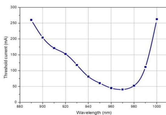
阈值电流
