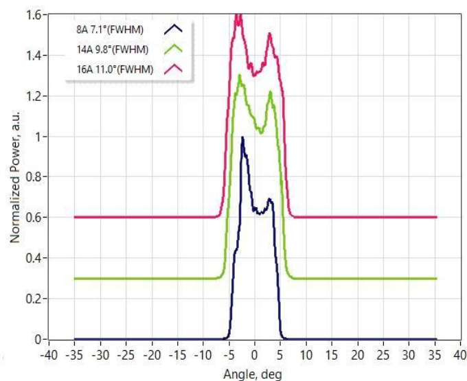
慢轴远场
