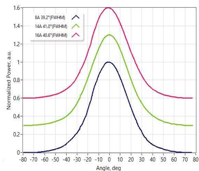
快轴远场
