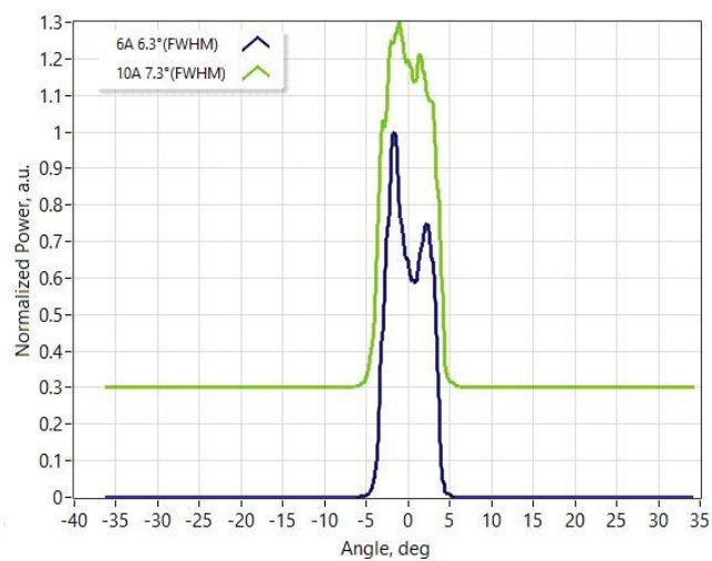
慢轴远场
