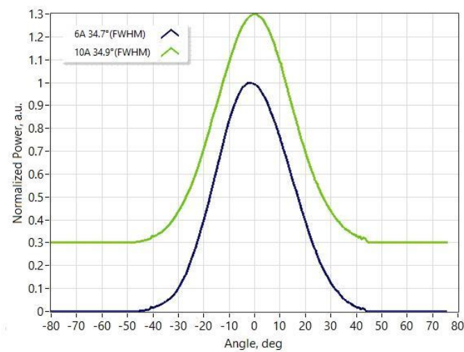
快轴远场
