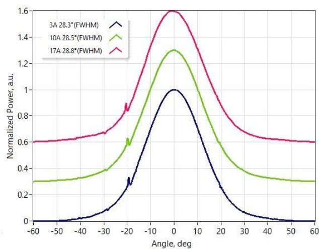
快轴远场
