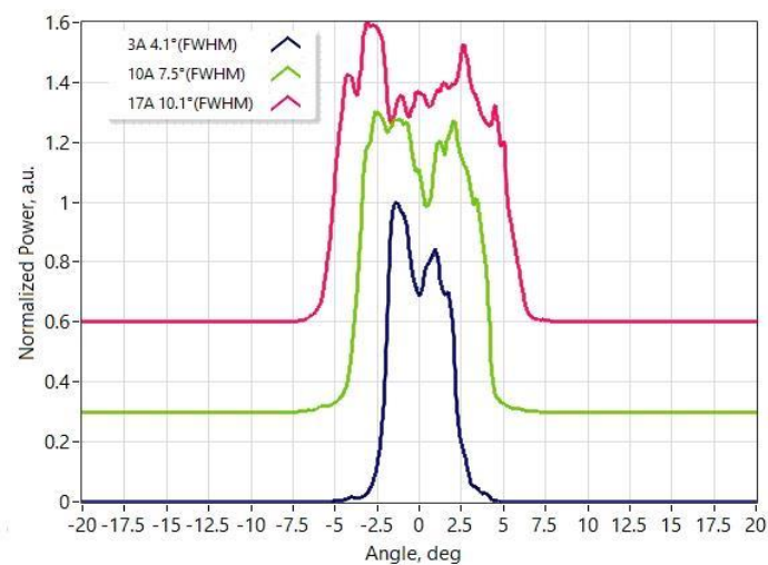
慢轴远场
