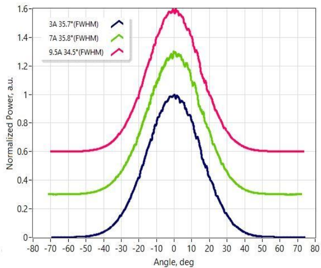
快轴远场
