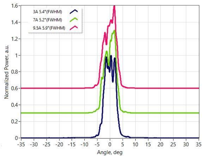
慢轴远场
