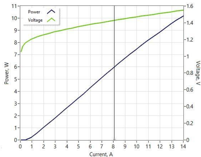
光-电流-电压特性
