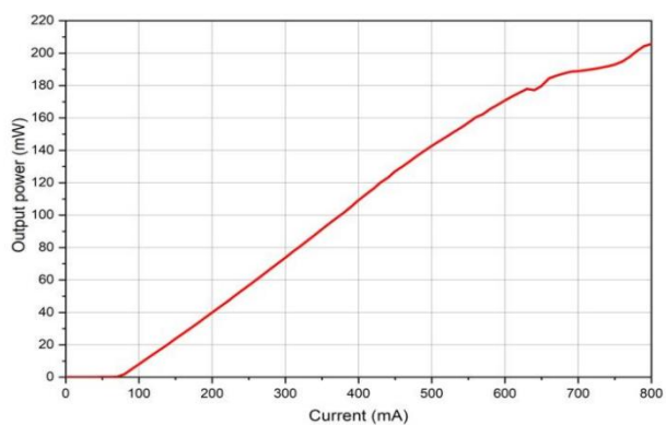
无反馈时的典型表现 (仅供参考)
