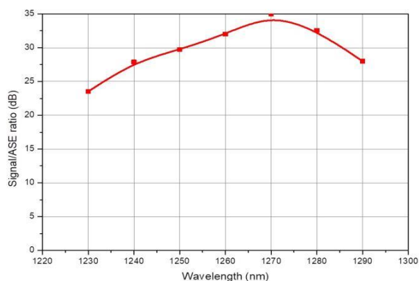
积分信号/ASE 比率
