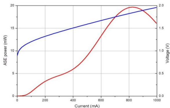
L-I-V 曲线
