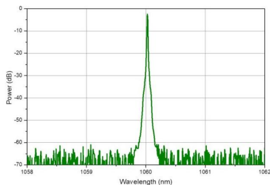
光谱(res. 10pm)
