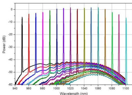
光谱(res. 0.5 nm)
