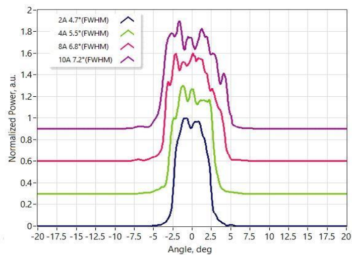
慢轴远场
