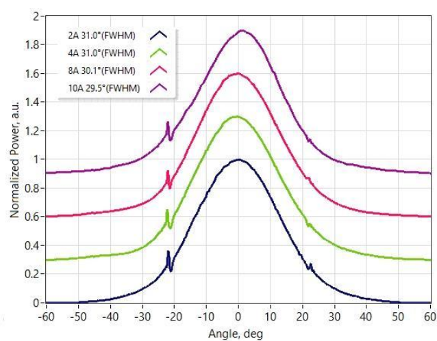
快轴远场
