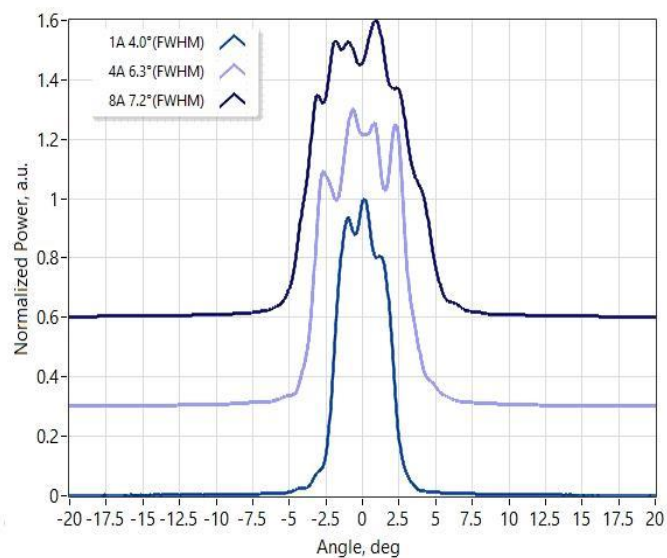
慢轴远场
