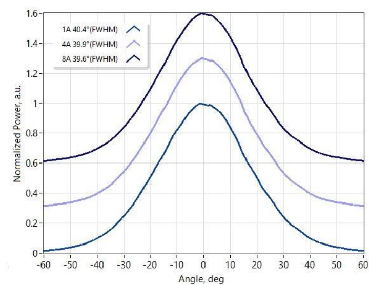
快轴远场
