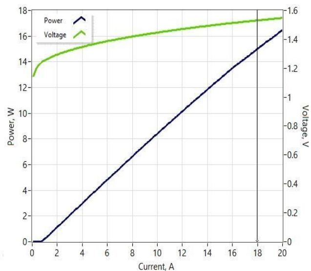
光-电流-电压特性
