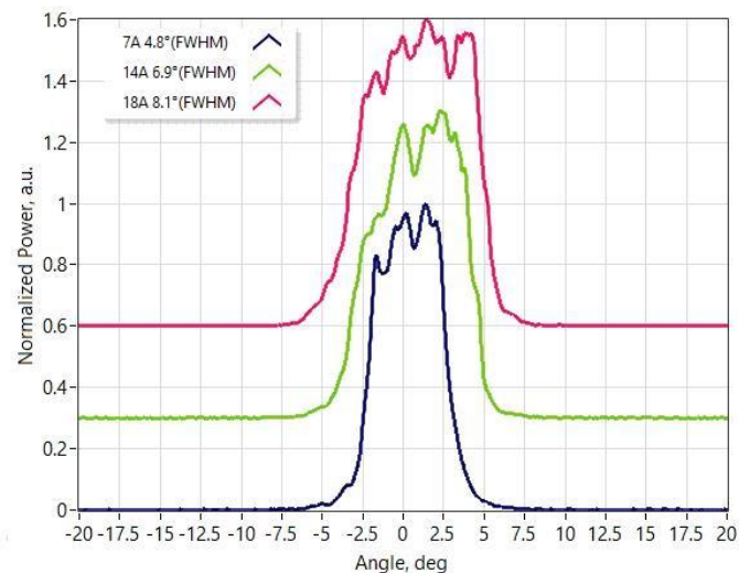
慢轴远场
