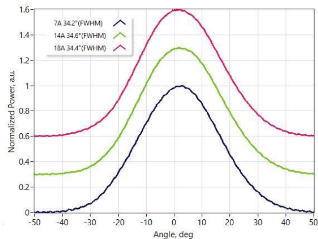
快轴远场
