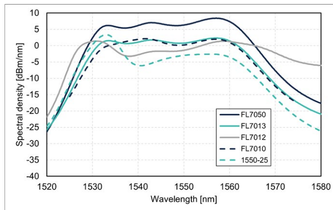
光谱密度与波长 (C波段)
