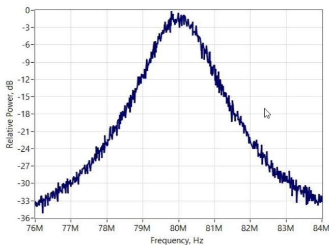
RF-line Spectrum
