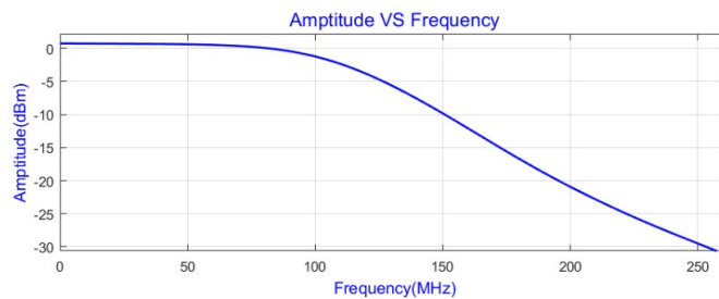
300MHz带宽相应曲线
