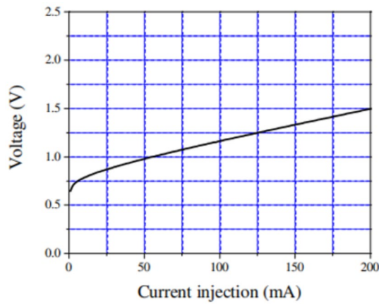
I-V 曲线
