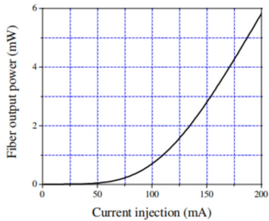
电流功率曲线
