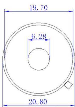
俯视图
